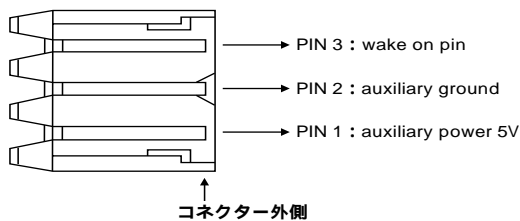
コネクターピンアサイン
